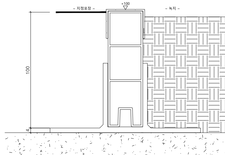
멀티엣지(W30) H100 단면도
