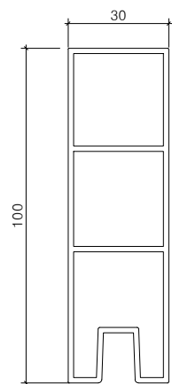
멀티엣지(W30) 알루미늄구조도(H100)
