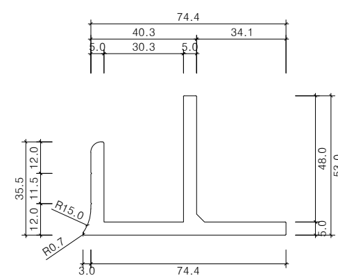
하부고정철물(W30) 상세도
