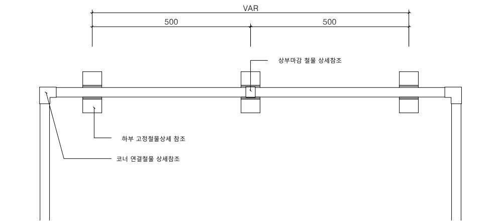
멀티엣지(W30) H100 평면도
